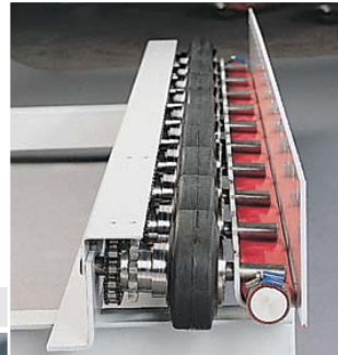
Rouleaux débrayables Declutching rollers
