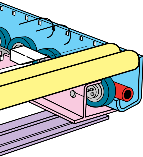
Cellule sous les rouleaux avec rouleau encoché Photocell under rollers with a notched roller
