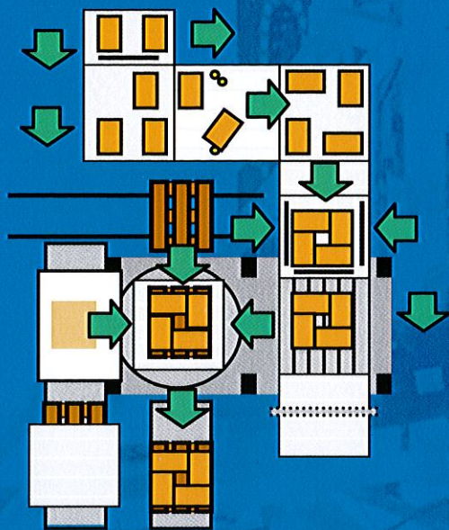
Palettisation en ligne avec un découpeur
