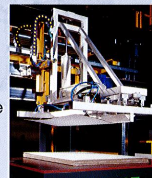
Inséreur d'intercalaire et de macule
