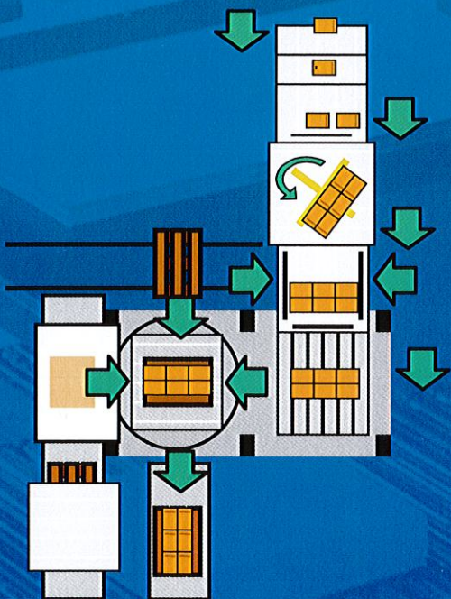
Palettisation en ligne avec un combiné
